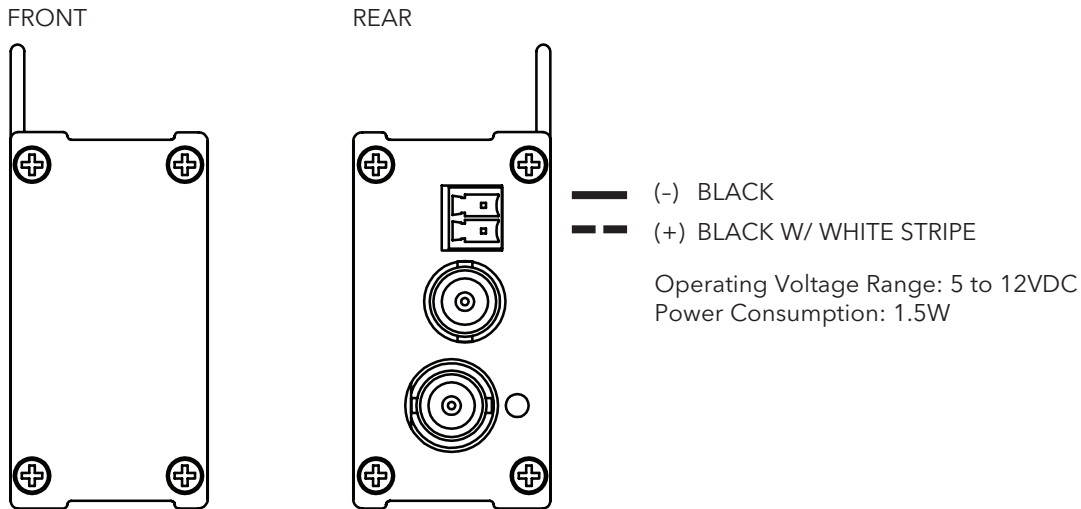
FIGURE 2 - FVT1/M MINI TRANSMITTER
