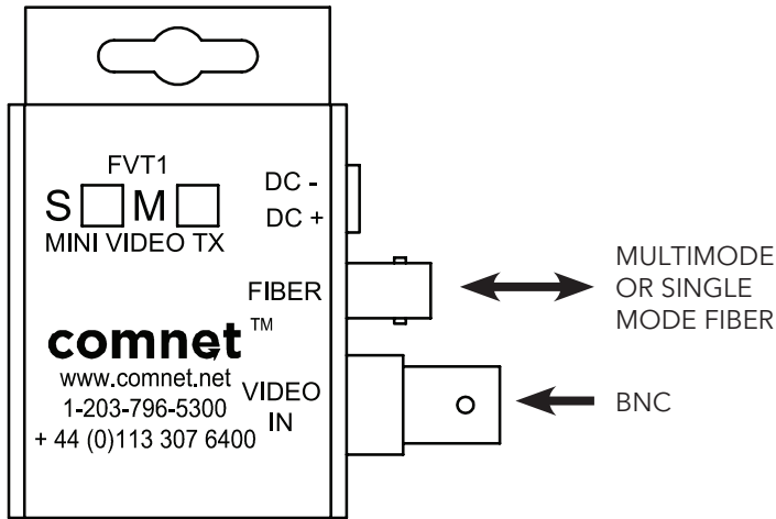
FIGURE 1 - FVT1/M MINI TRANSMITTER
